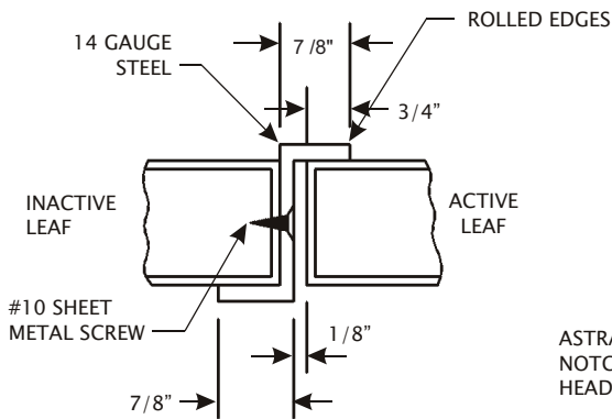
'Z' ASTRAGAL
